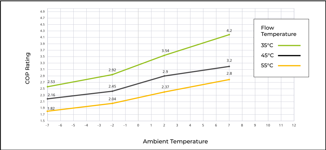
ECOMOD 32kW
