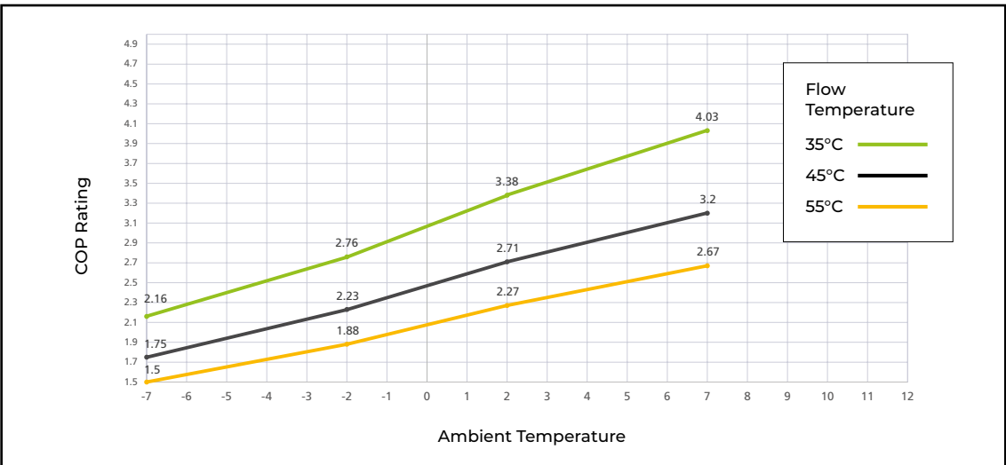
ECOMOD 50kW
