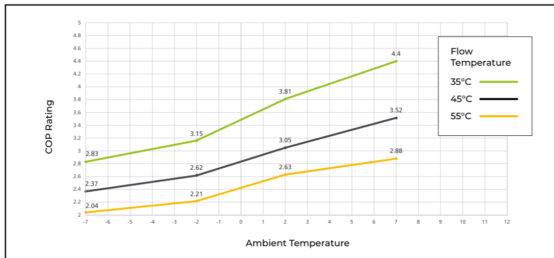
ECOMOD 18kW
