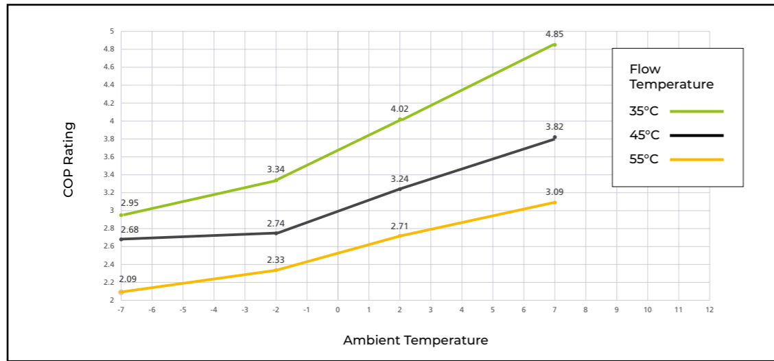
ECOMOD 14kW
