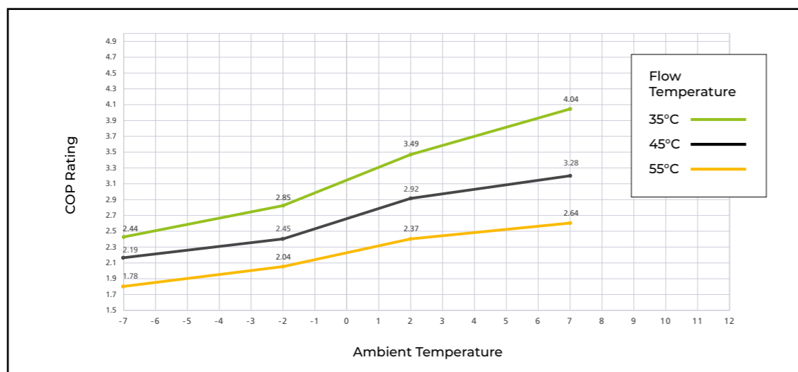
ECOMOD 26kW
