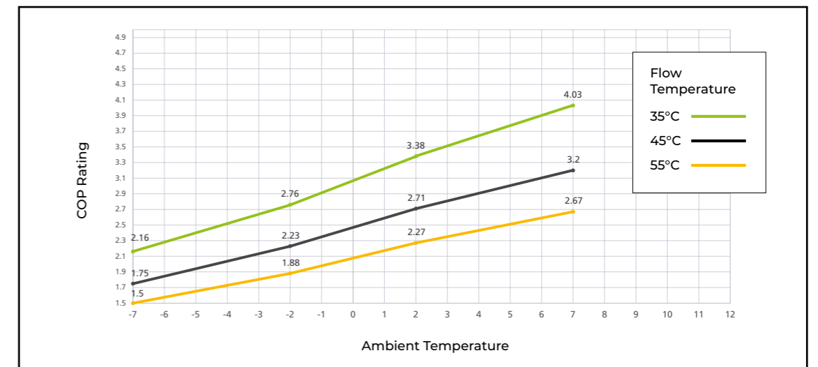
ECOMOD 50kW
